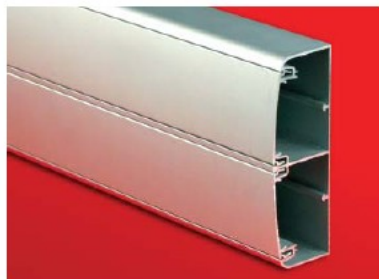
Алюминиевый кабель-канал 140x50 мм со встроенным разделителем и двумя крышками. Длина 2 метра
